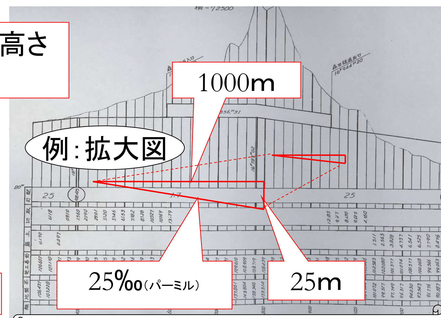
縦断面図(「土木構造物保守台帳」より)
