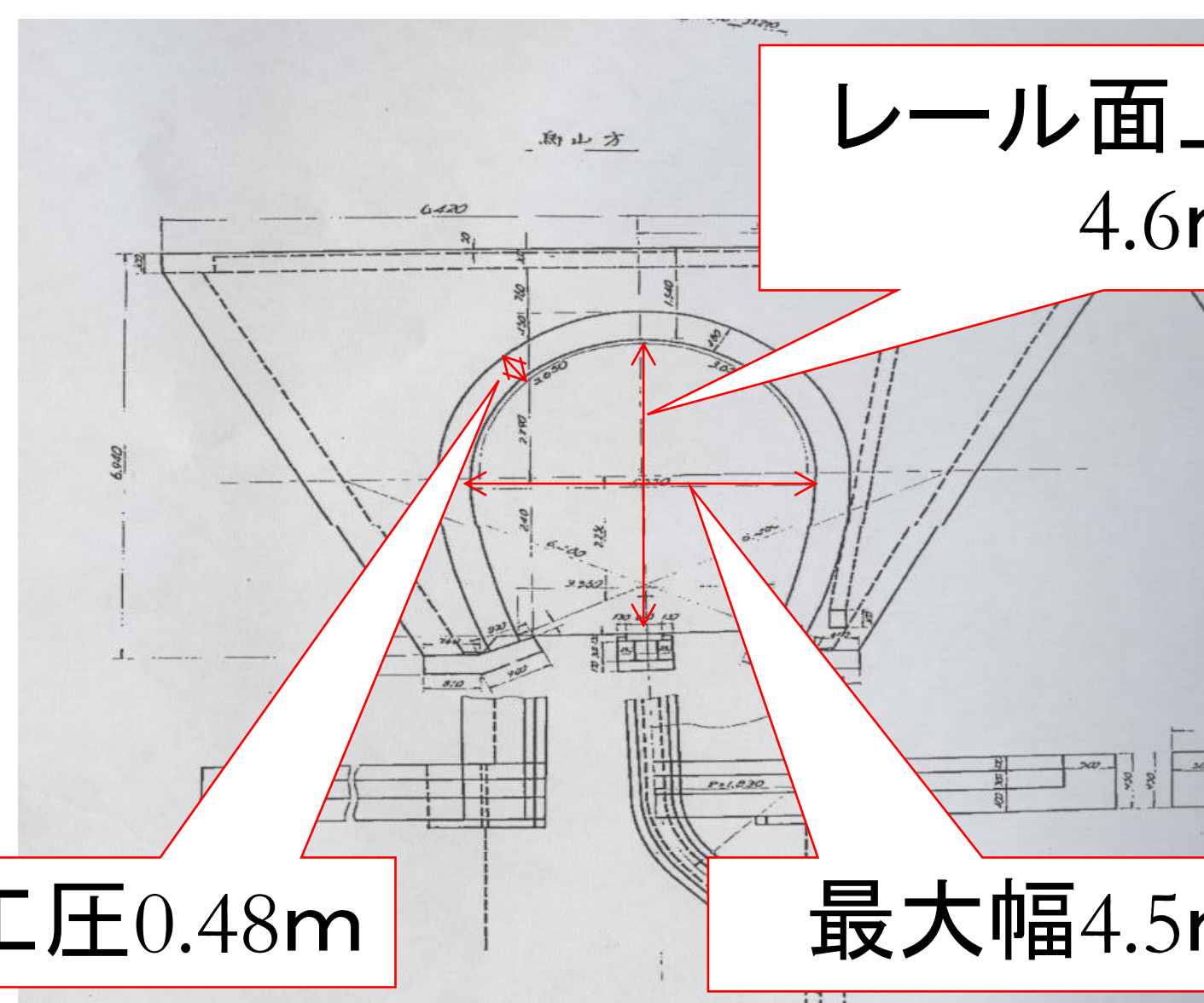
横断面図(「土木構造物保守台帳」より)
