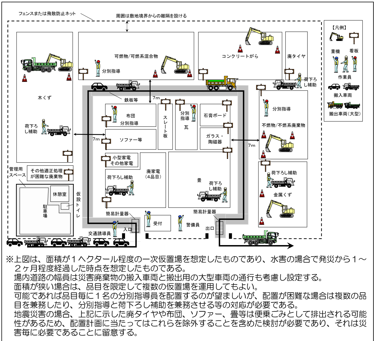
図表38 一次仮置場の配置計画（レイアウト）例
