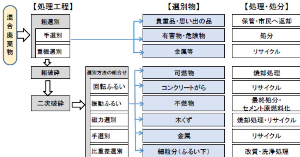
図表42 混合廃棄物の処理（例）
