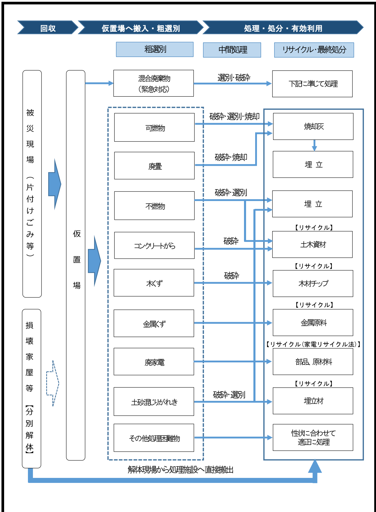
図表 4.5 災害廃棄物の処理フロー
