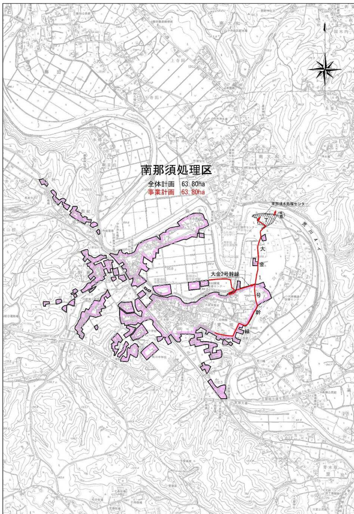
図 2.2.2 公共下水道事業計画一般図（南那須処理区）
