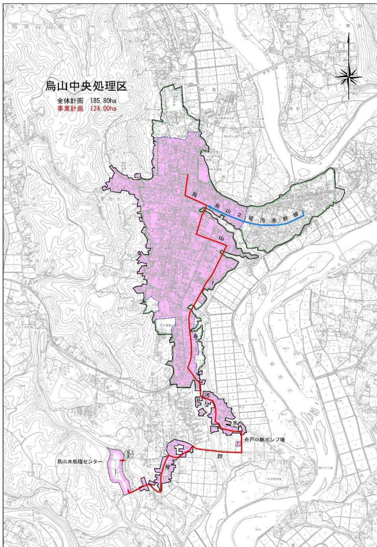
図 2.2.1 公共下水道事業計画一般図（烏山中央処理区）
